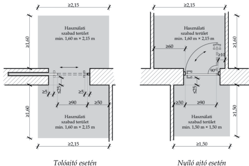
AKADÁLYMENTES AJTÓBEÉPÍTÉS ÉS HASZNÁLATI SZABAD TERÜLET MINIMÁLIS MÉRETE
